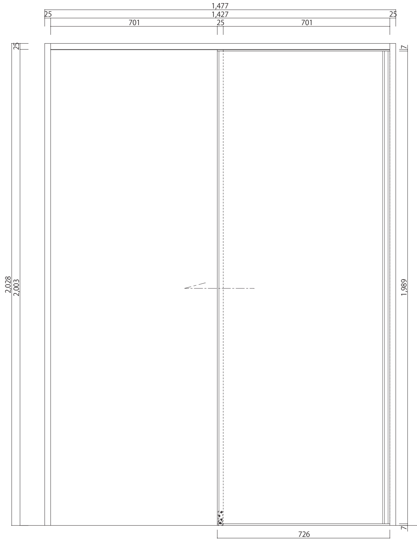
【建具正面図】
