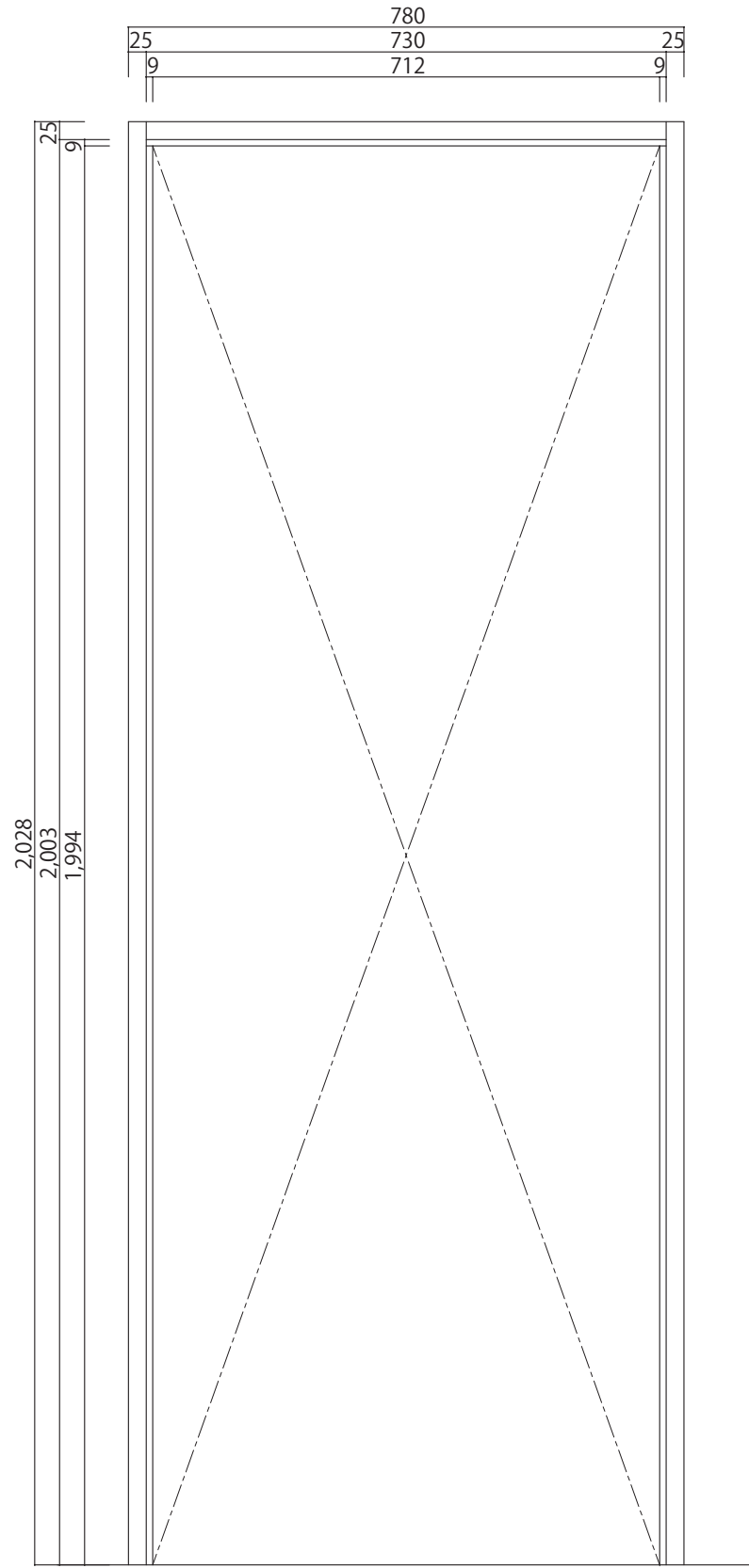
【枠正面図】
