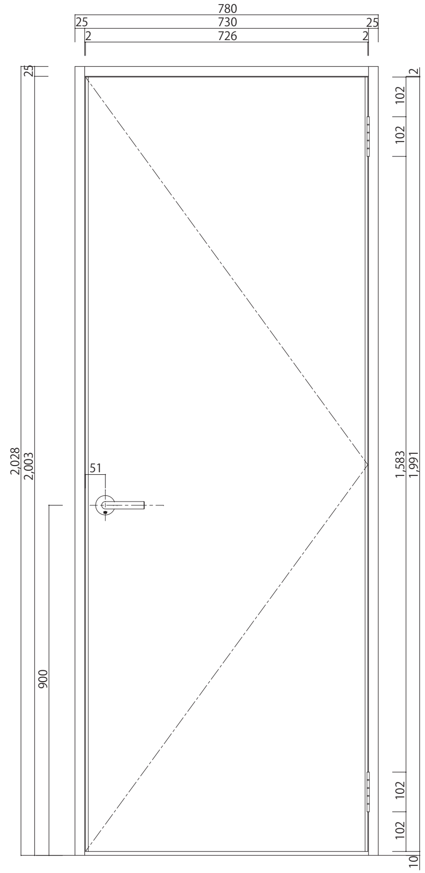
【建具正面図】
